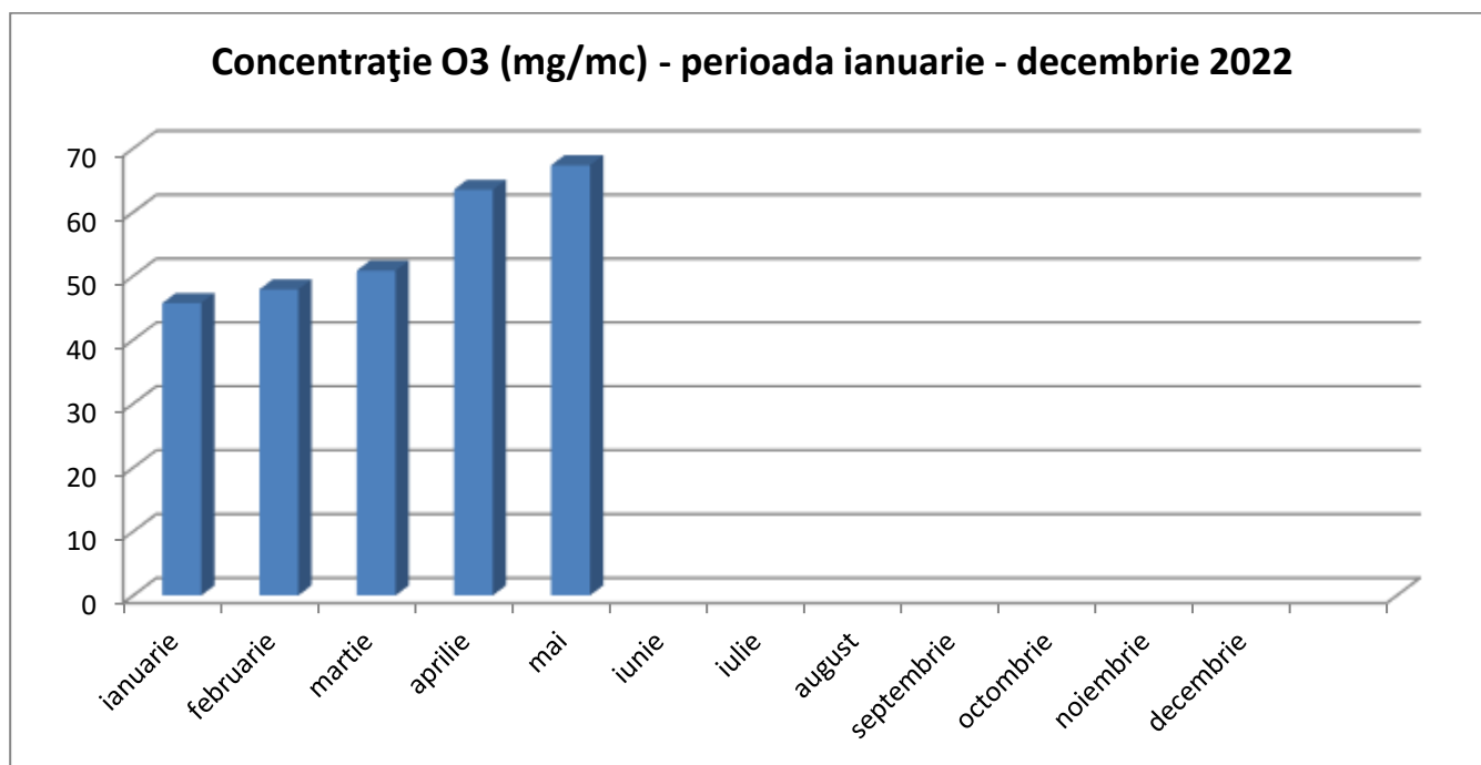
Fig. I.1.1.4.1. Ozonul (O 3 ) - valori medii lunare 2022, stația OT1
