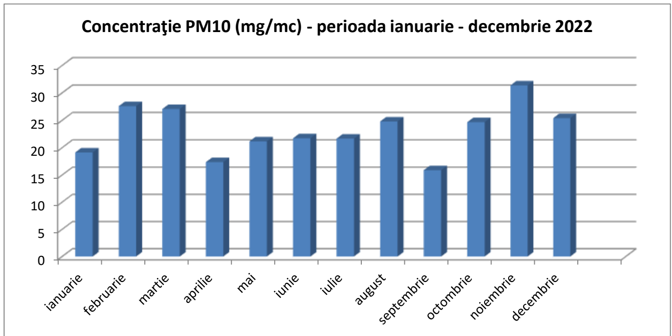
Fig. I.1.1.5.2 Particule în suspensie (PM10) - concentrații medii lunare 2022
