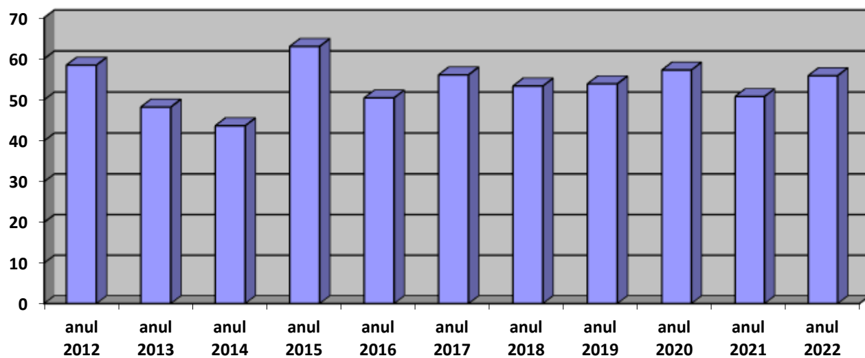
Fig. I.1.1.2.4. Evoluția concentrației medii anuale de ozon ( \mu\text{g}/\text{mc} )
