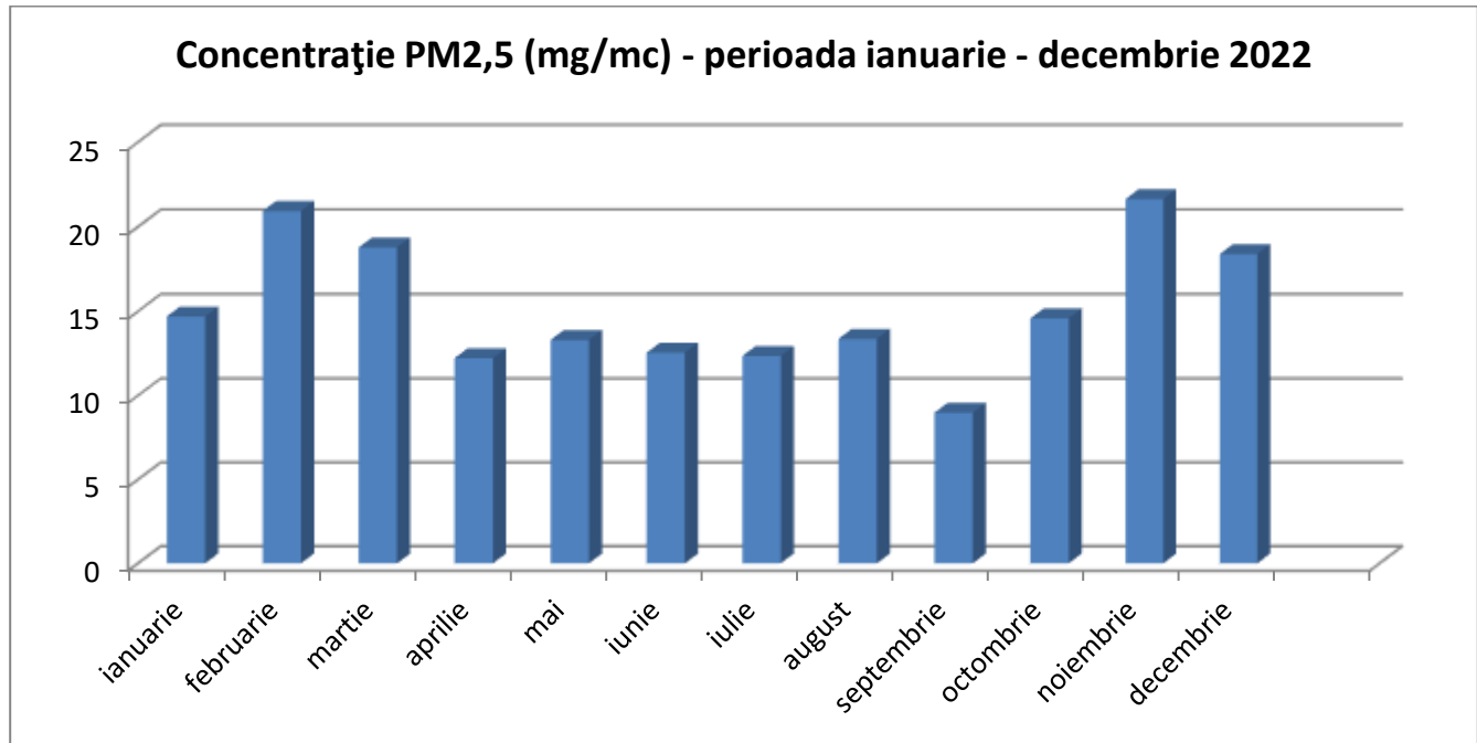
Fig. I.1.1.1.6. Particule în suspensie (PM 2,5 ) - concentrații medii lunare 2022
