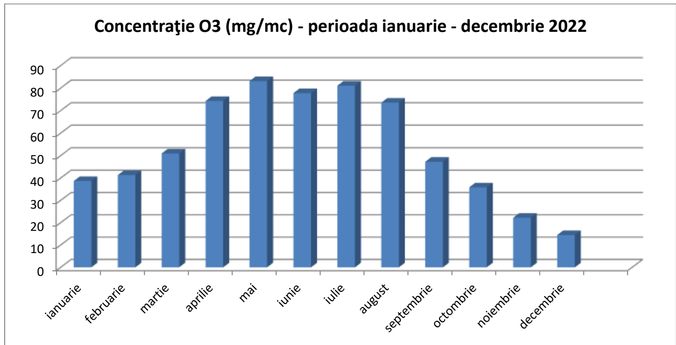
Fig. I.1.1.1.4.2. Ozonul (O 3 ) - valori medii lunare 2022, stația OT2
