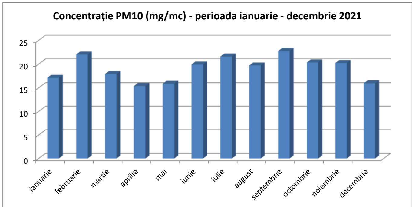
Fig. I.1.1.1.5. Particule în suspensie (PM10) - concentrații medii lunare 2021
