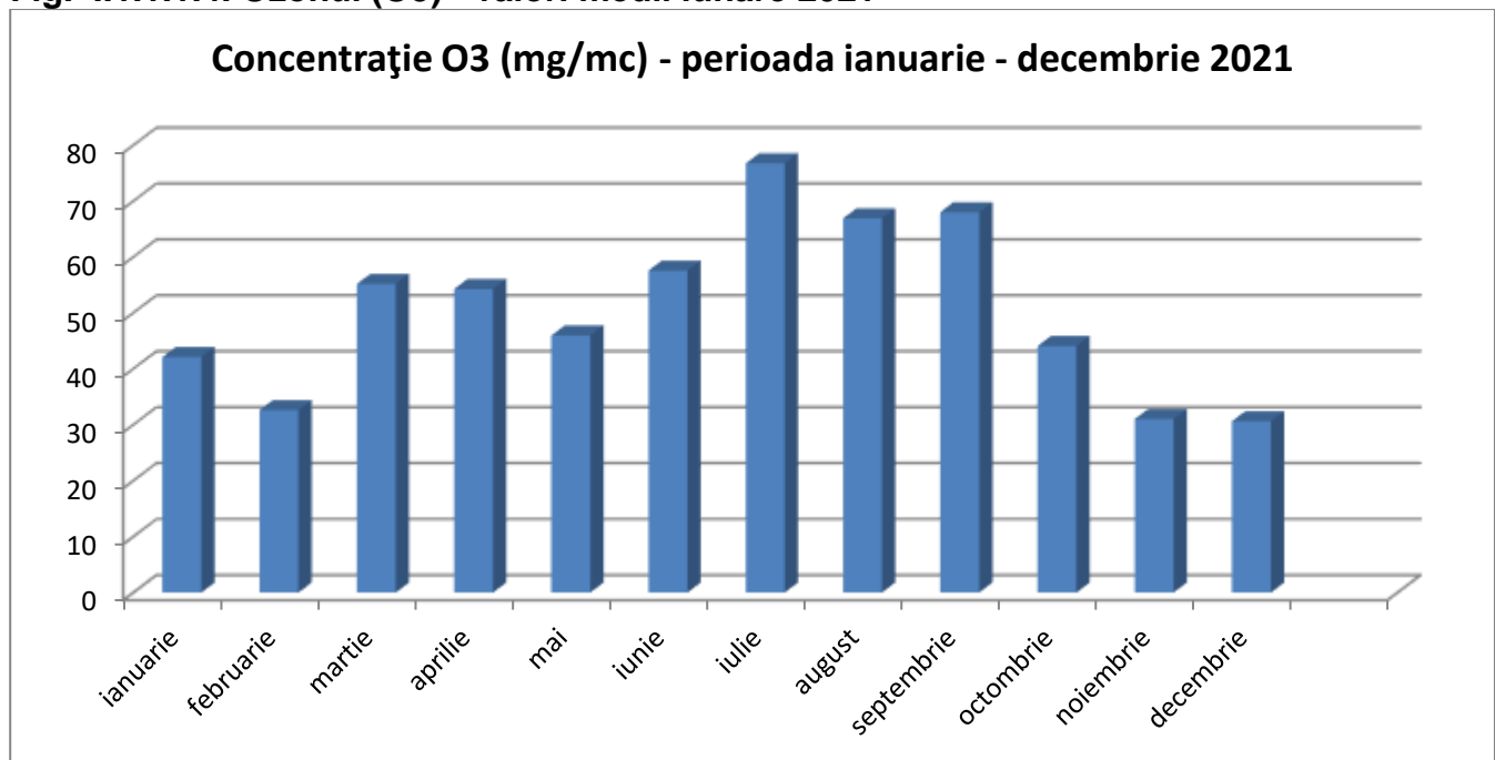
Fig. I.1.1.1.4. Ozonul (O 3 ) - valori medii lunare 2021
