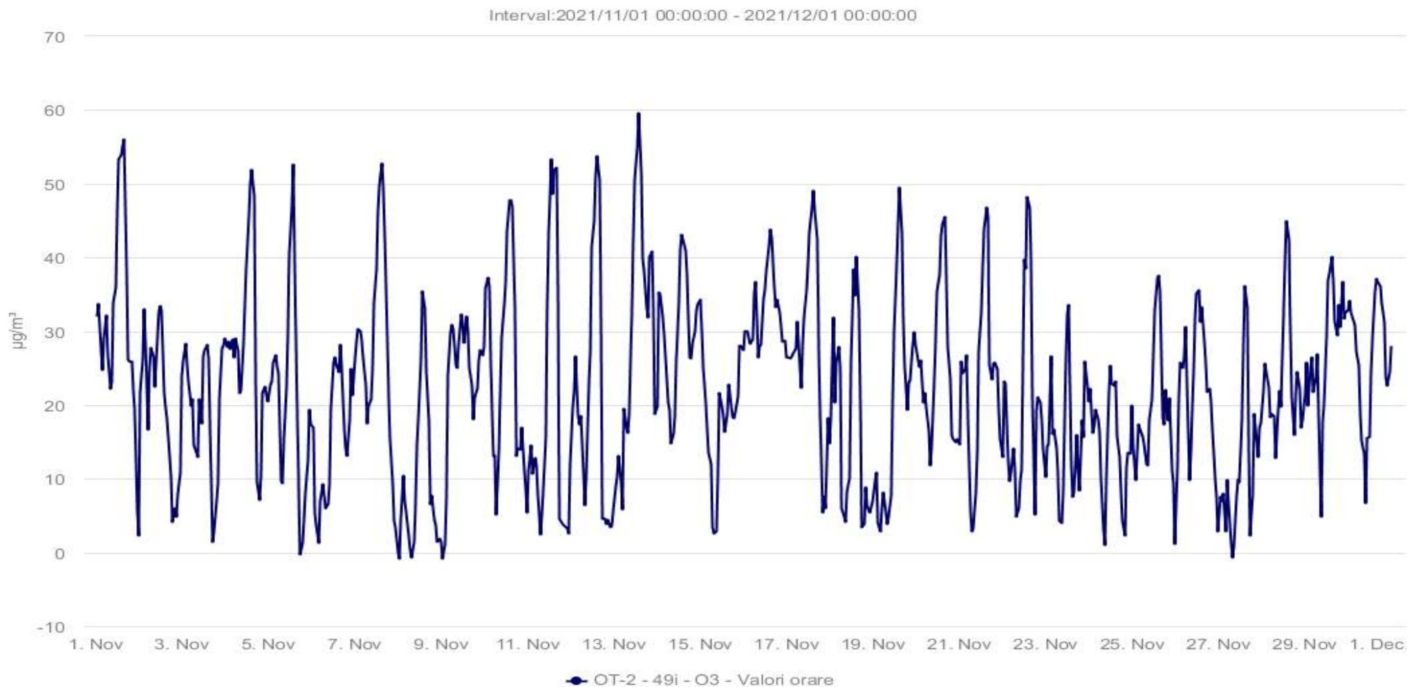
Fig. 1.8 Evoluție valori medii orare pentru O_3 - luna NOIEMBRIE 2021
