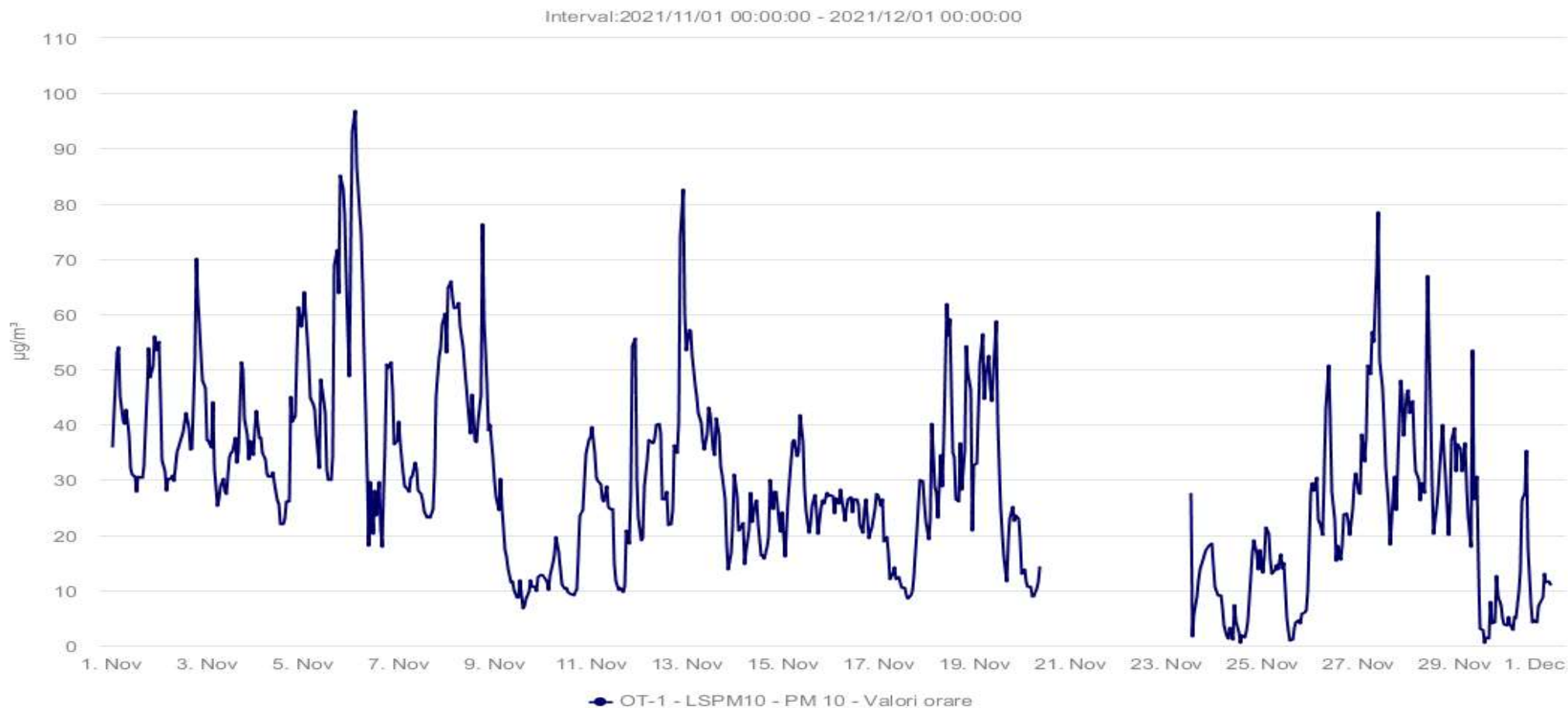
Fig. 1.6 Evoluție valori medii orare PM10 la stația automată din județul Olt – luna NOIEMBRIE 2021
