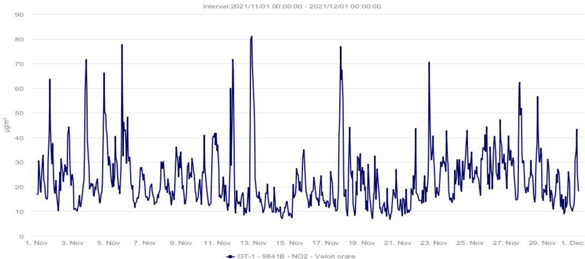
Fig. 1.5 Evoluție valori medii orare NO 2 la stația automată din județul Olt – luna NOIEMBRIE 2021
