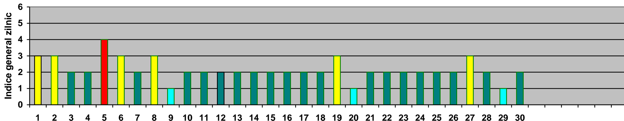
Fig.1.2. Evoluția indicelui general de calitate a aerului în luna NOIEMBRIE 2021 la stația OT-1 (Slatina, Aleea Grădiște F.N.)
