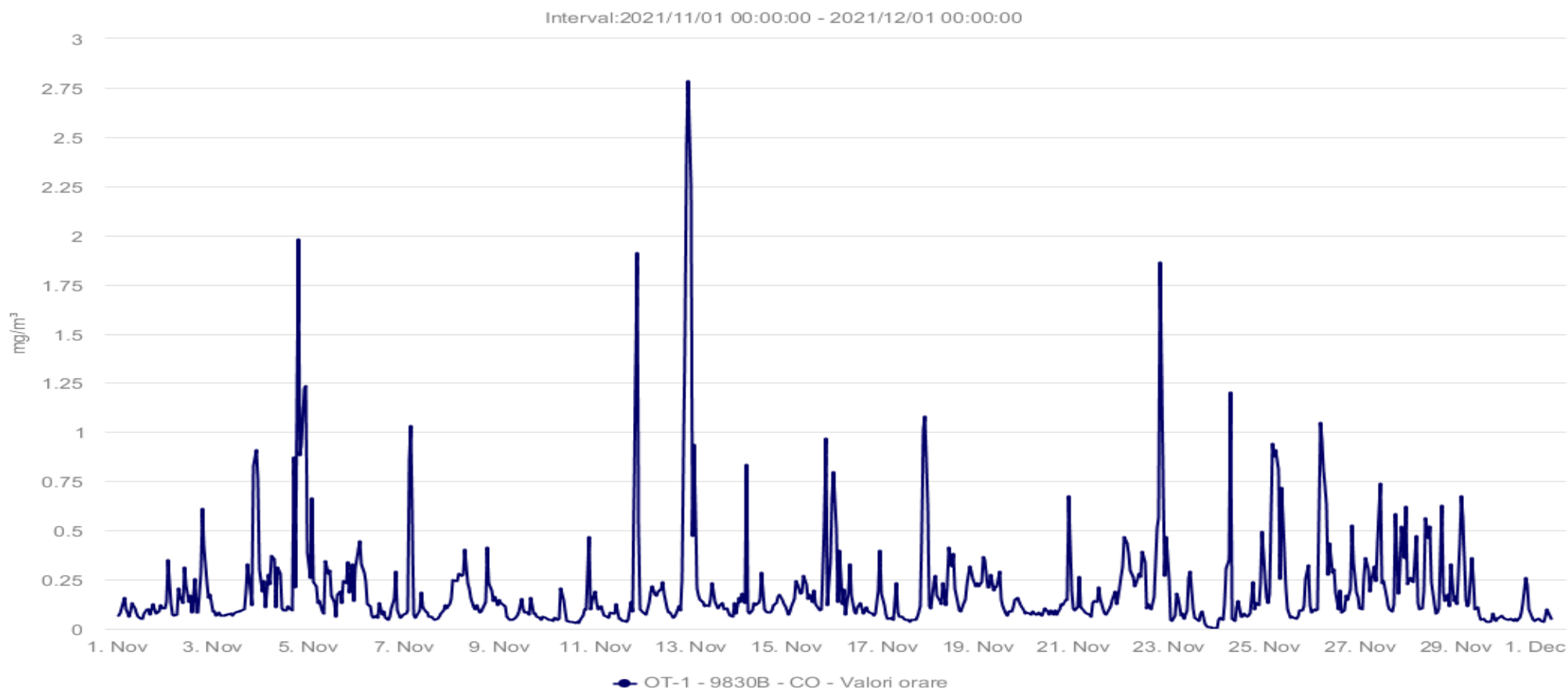
Fig. 1.7 Evoluție valori medii orare pentru CO - luna NOIEMBRIE 2021
