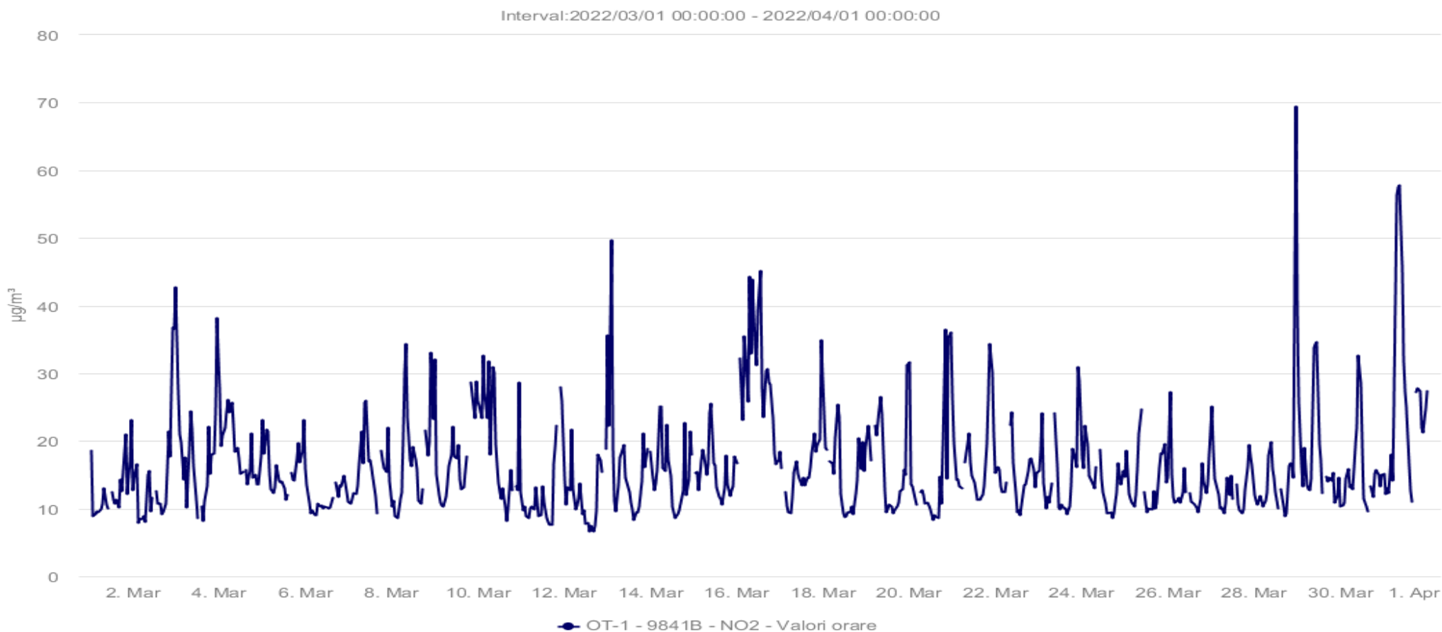
Fig. 1.5 Evoluție valori medii orare NO 2 la stația automată din județul Olt – luna MARTIE 2022
