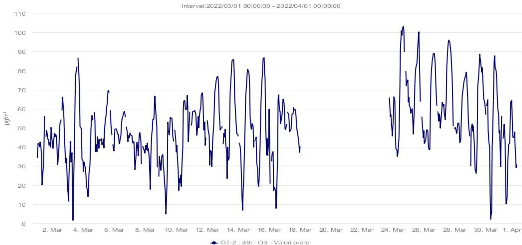
Fig. 1.8 Evoluție valori medii orare pentru O_3 - luna MARTIE 2022
