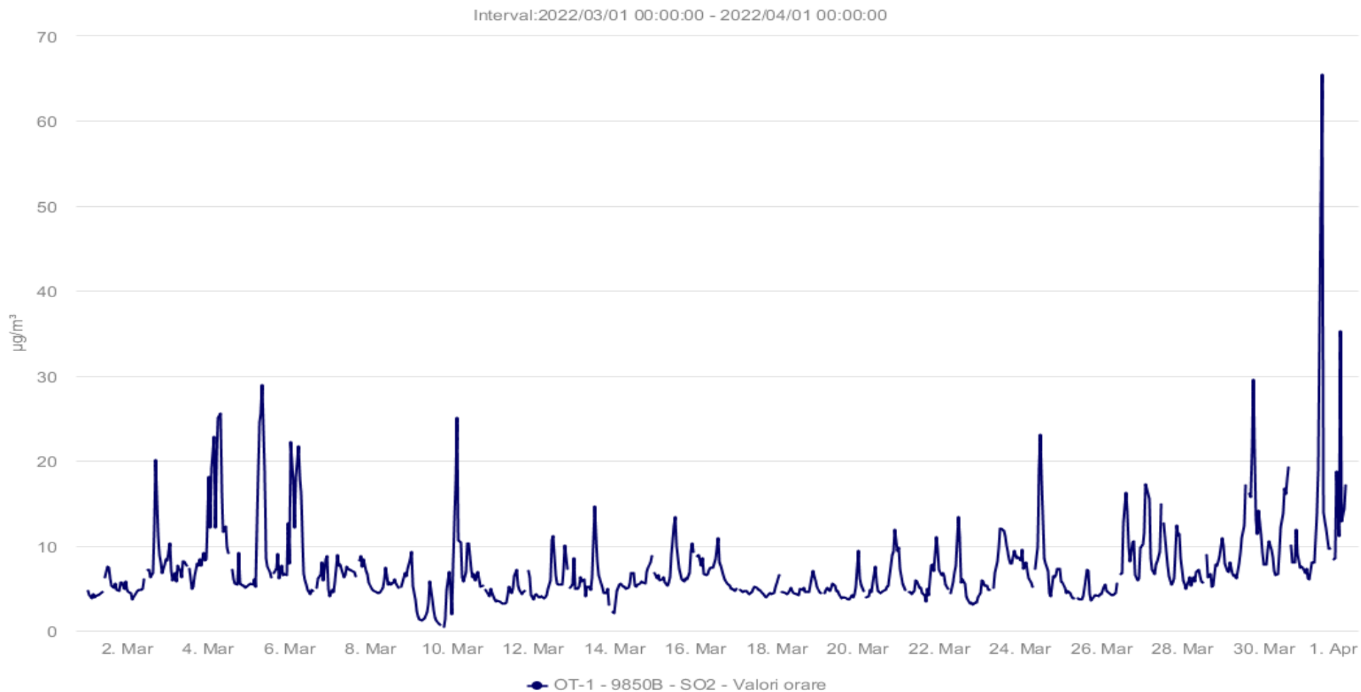
Fig. 1.4 Evoluție valori medii orare SO 2 la stația automată OT1 din județul Olt – luna MARTIE 2022.
