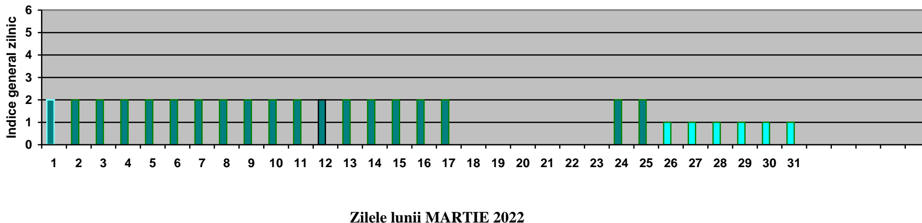
Fig.1.3 Evoluția indicelui zilnic general de calitate a aerului în luna MARTIE 2022 la stația OT-2 (Slatina, Aleea Muncii, nr 4)
