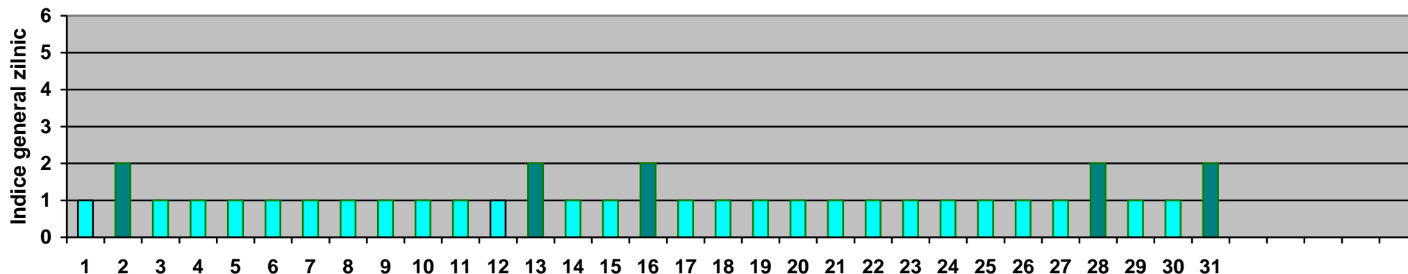
Fig.1.2. Evoluția indicelui general de calitate a aerului în luna MARTIE 2022 la stația OT-1 (Slatina, Aleea Grădiște F.N.)
