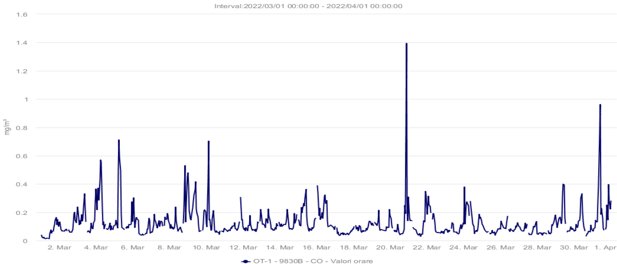
Fig. 1.7 Evoluție valori medii orare pentru CO - luna MARTIE 2022
