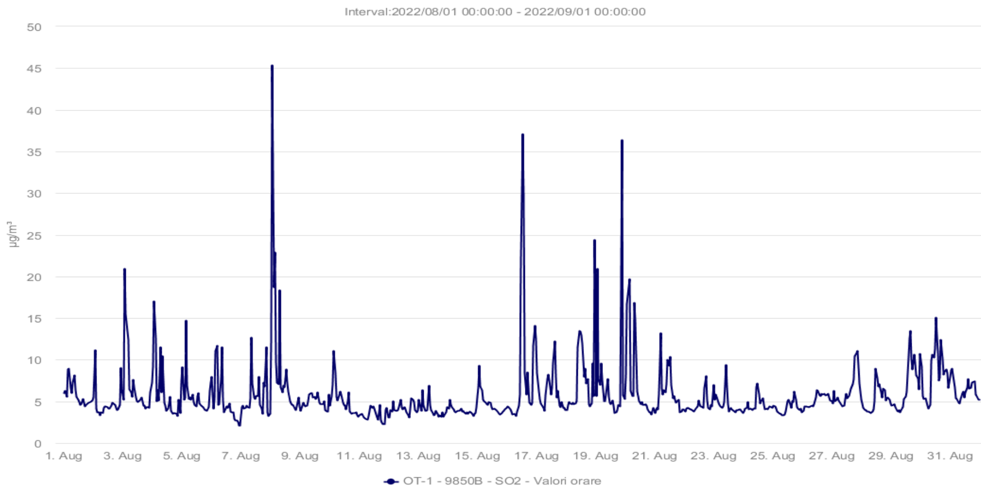
Fig. 1.4 Evoluție valori medii orare SO 2 la stația automată OT1 din județul Olt – luna AUGUST 2022.
