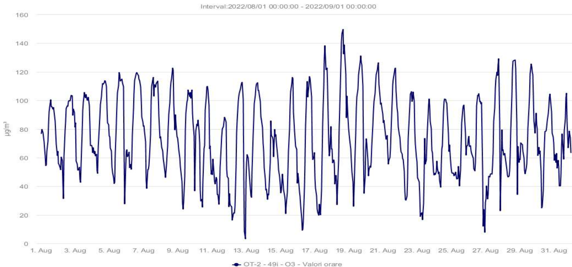
Fig. 1.6 Evoluție valori medii orare pentru O_3 - luna AUGUST2022
