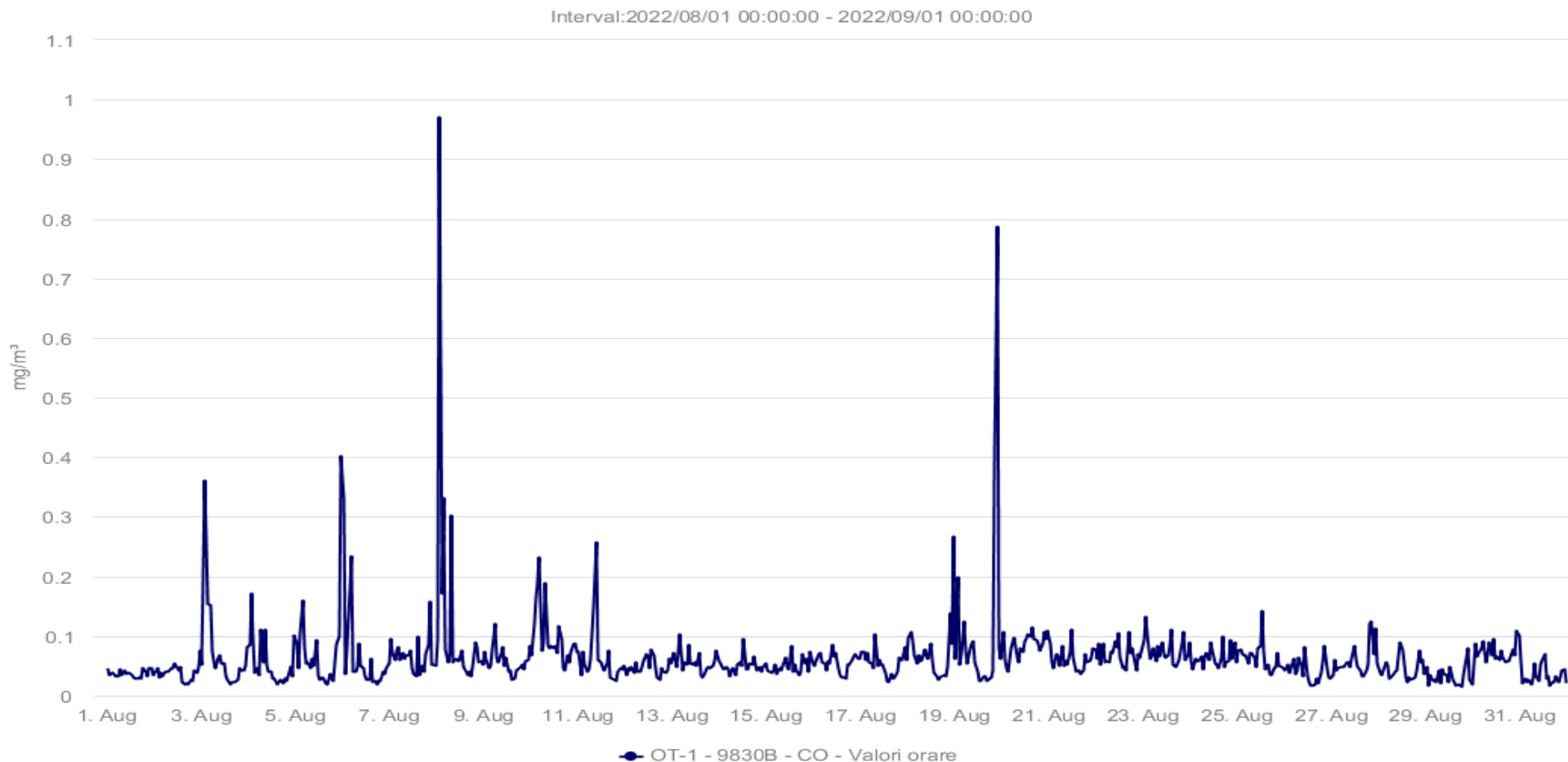
Fig. 1.5 Evoluție valori medii orare pentru CO - luna AUGUST 2022
