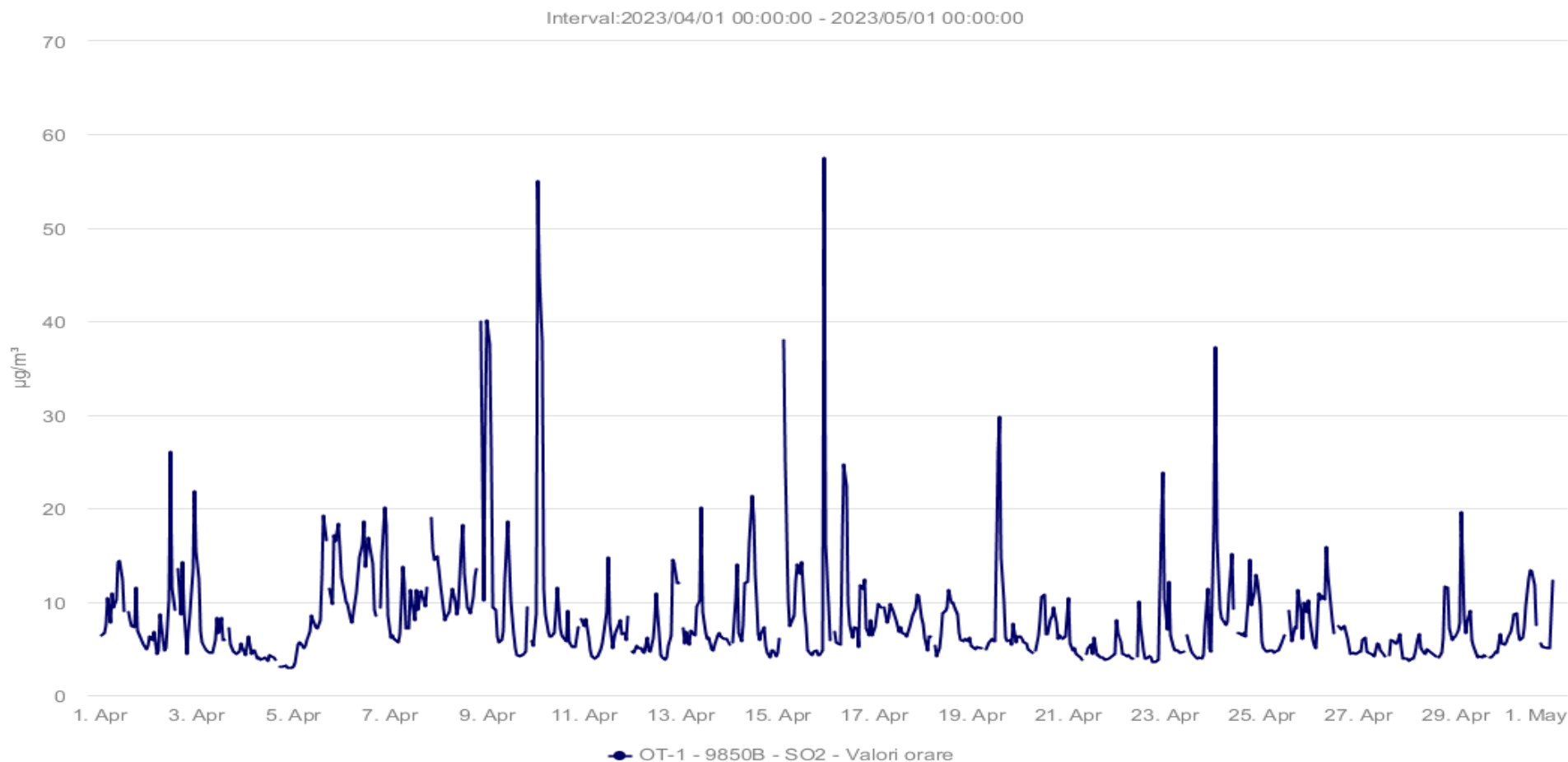
Fig. 1.4 Evoluție valori medii orare SO 2 la stația automata OT1 din județul Olt – luna APRILIE 2023.
