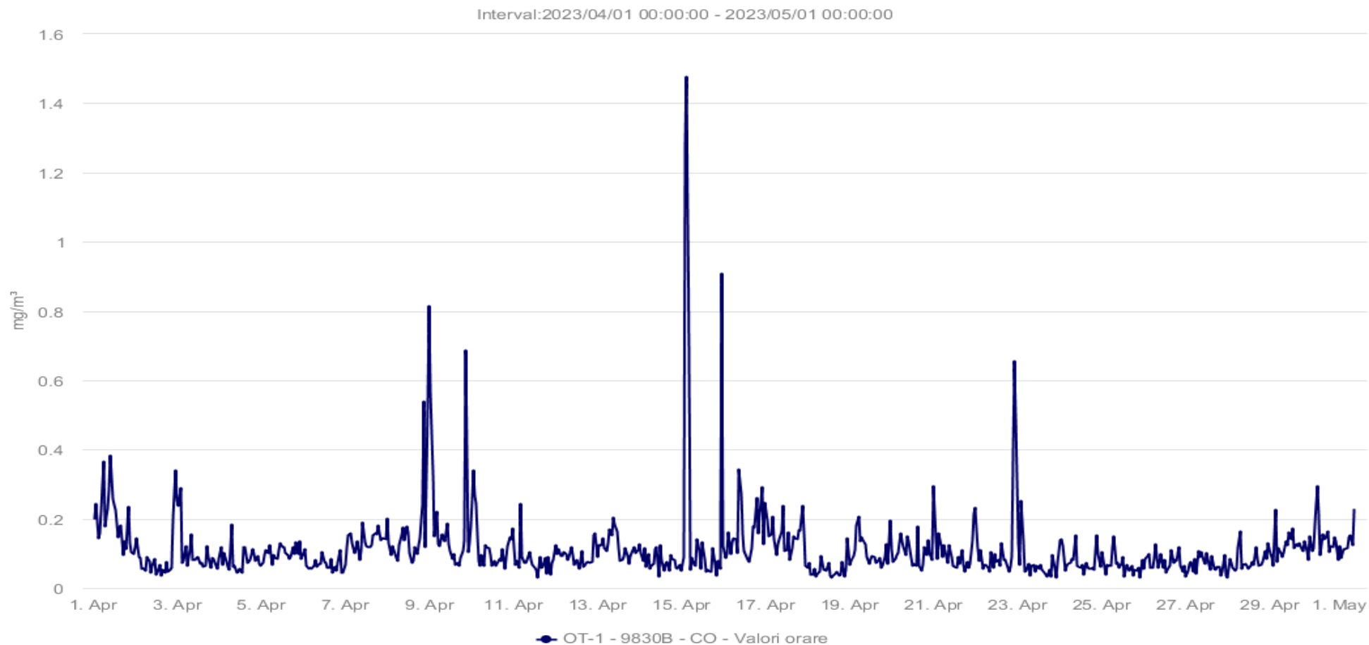
Fig. 1.5 Evoluție valori medii orare pentru CO - luna APRILIE 2023
