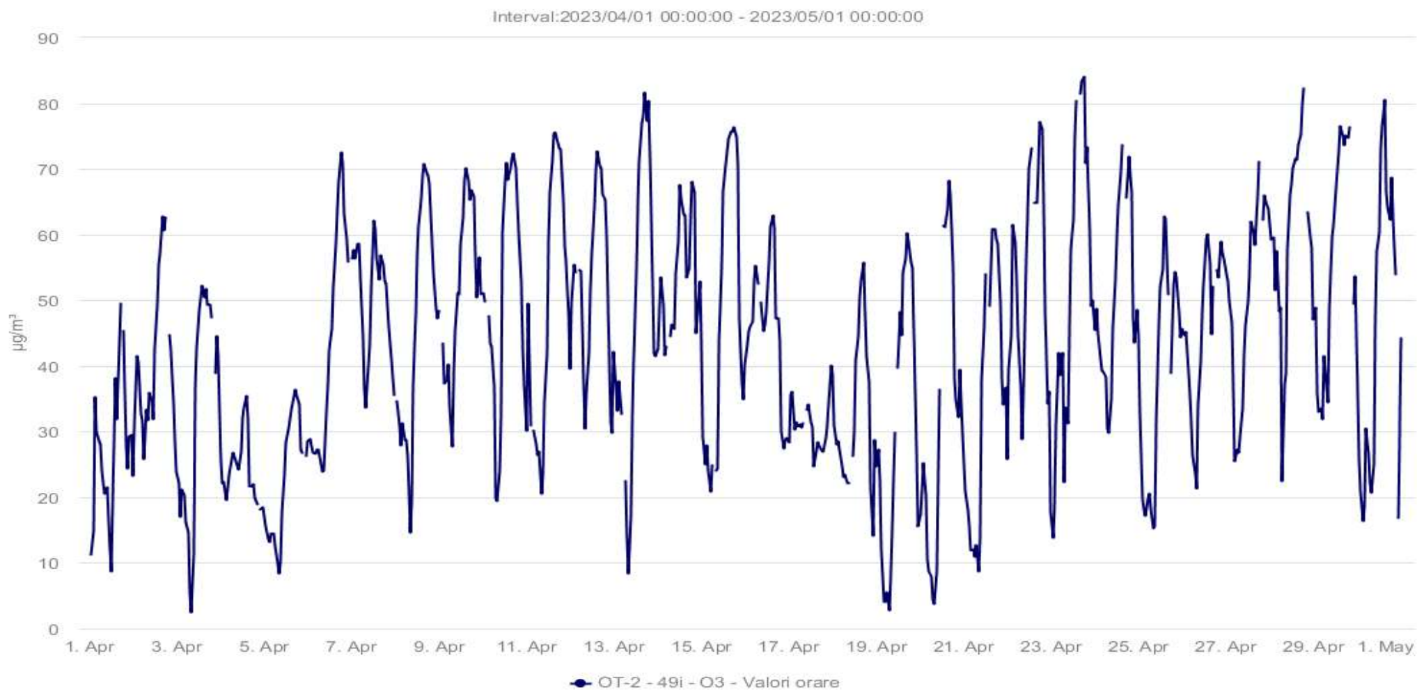
Fig. 1.7. Evoluție valori medii orare pentru O_3 - luna APRILIE 2023
