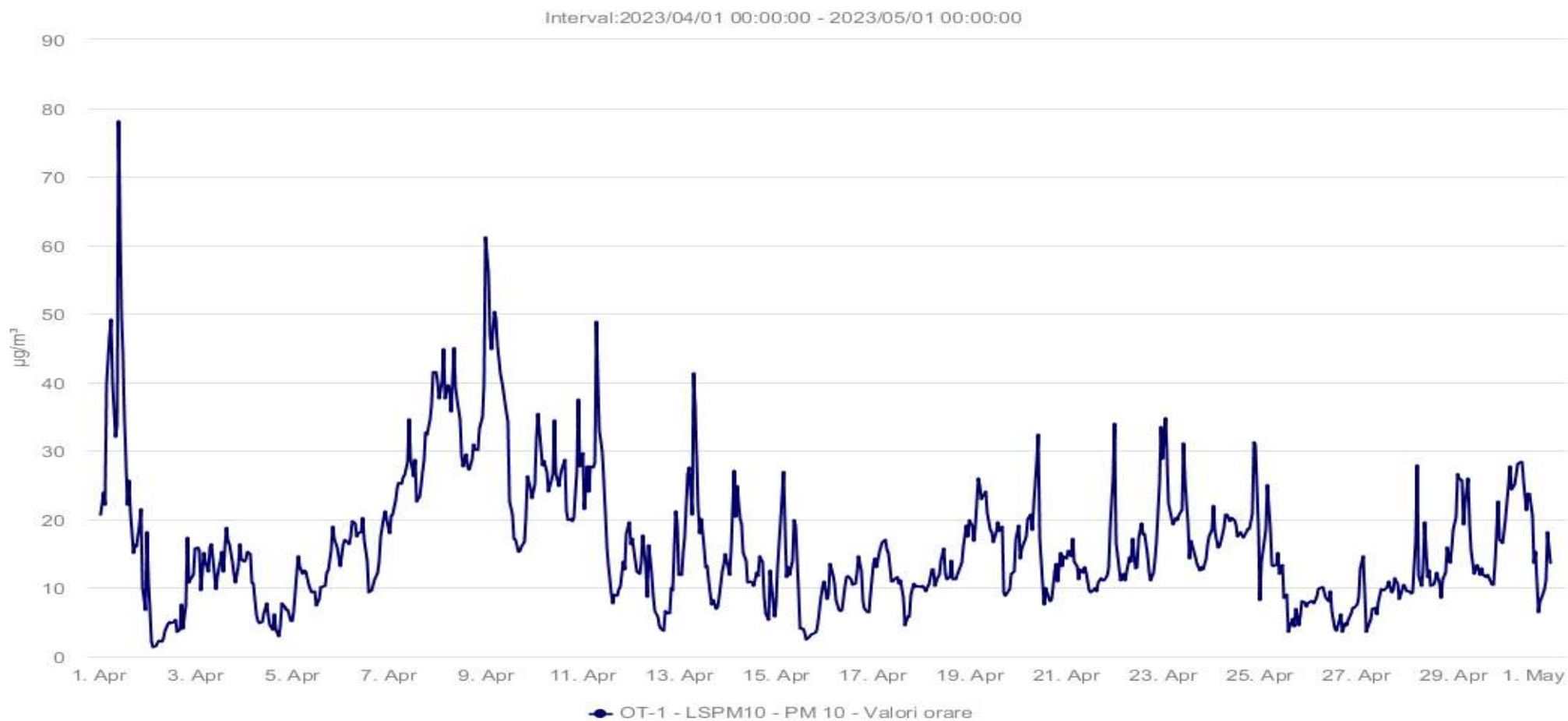
Fig. 1.6 Evoluție valori medii orare PM10 la stația automată din județul Olt – luna APRILIE 2023
