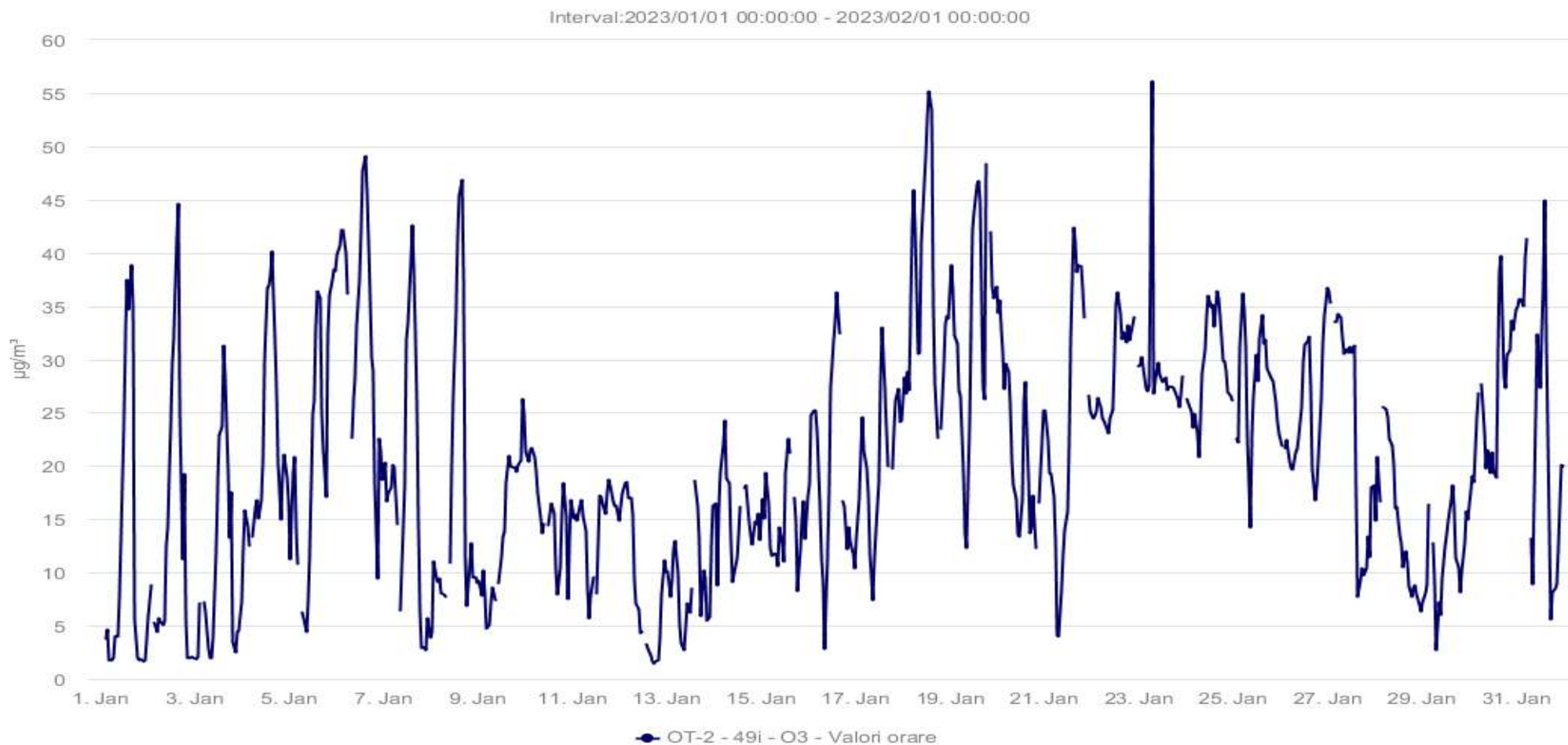
Fig. 1.7. Evoluție valori medii orare pentru O_3 - luna IANUARIE 2023
