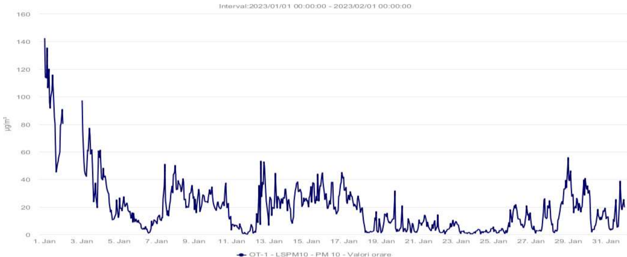
Fig. 1.6 Evoluție valori medii orare PM10 la stația automată din județul Olt – luna IANUARIE 2023
