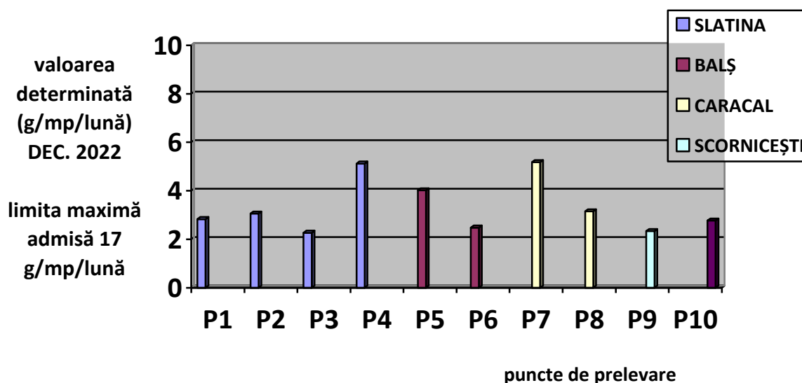
Fig. 1.8. Valori determinate pulberi sedimentabile
