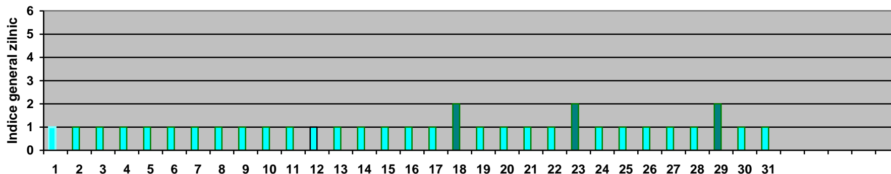
Fig.1.3 Evoluția indicelui zilnic general de calitate a aerului în luna IANUARIE 2023 la stația OT-2 (Slatina, Aleea Muncii, nr 4)
