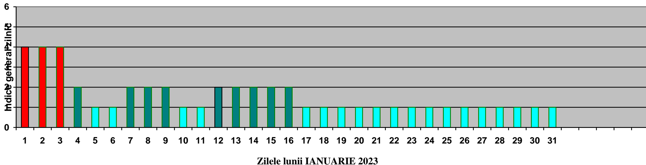
Fig.1.2. Evoluția indicelui general de calitate a aerului în luna IANUARIE 2023 la stația OT-1 (Slatina, Aleea Grădiște F.N.)
