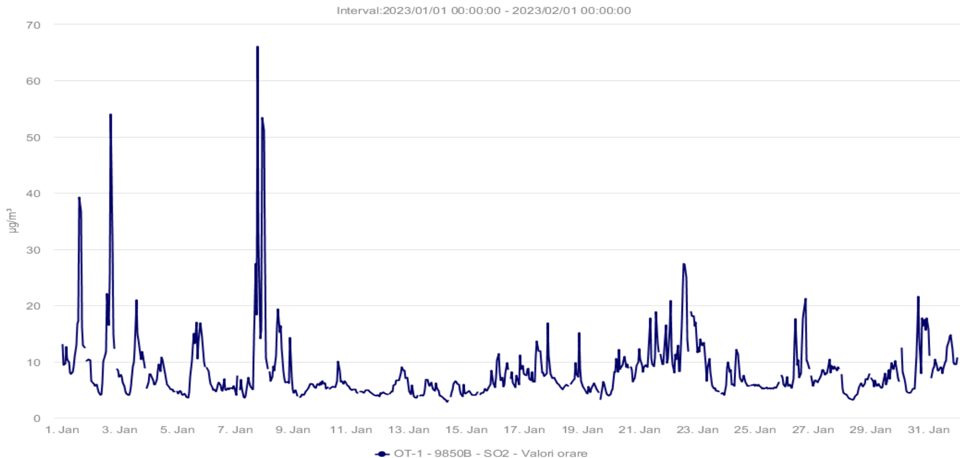
Fig. 1.4 Evoluție valori medii orare SO 2 la stația automată OT1 din județul Olt – luna IANUARIE 2023.
