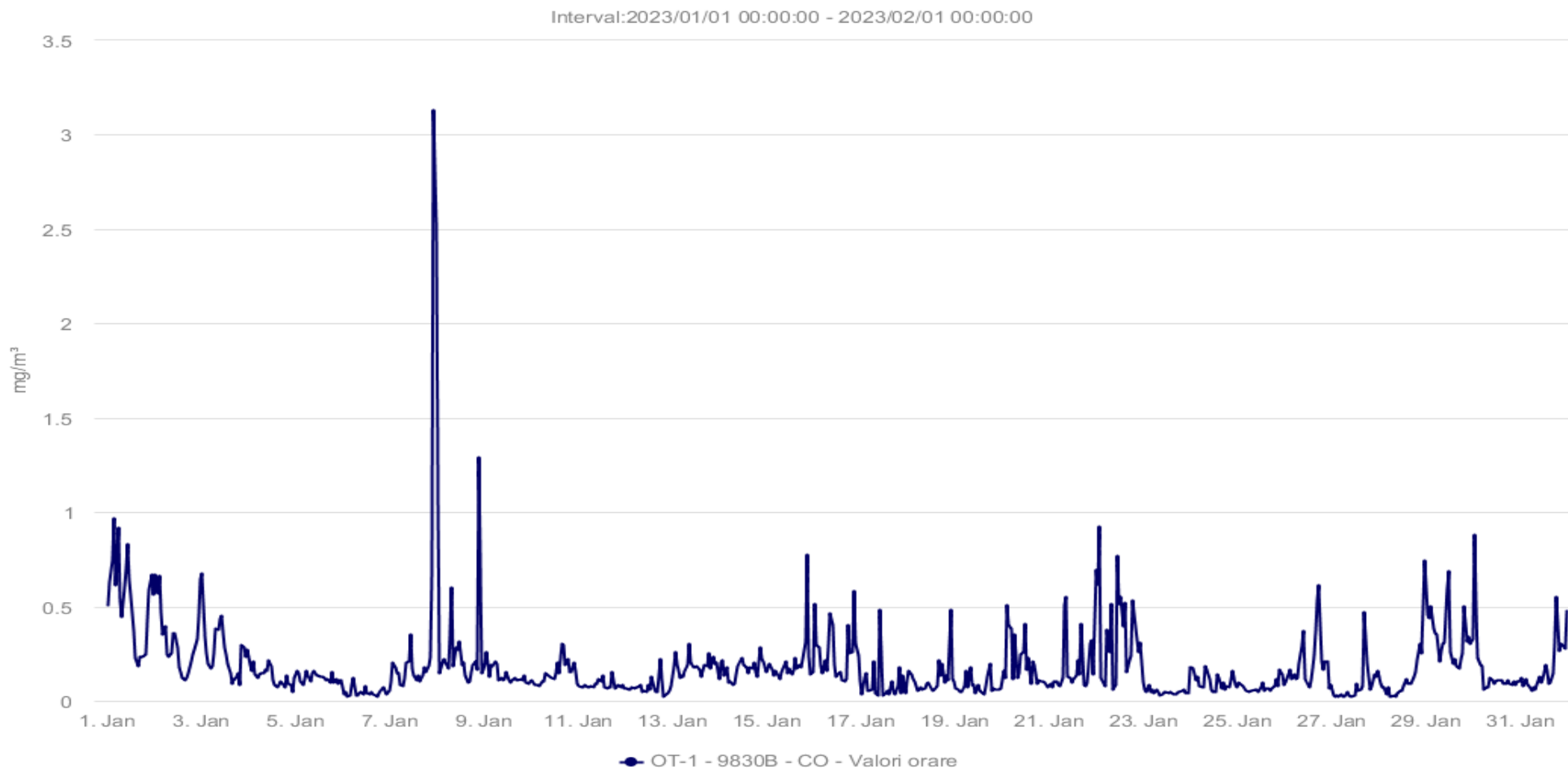
Fig. 1.5 Evoluție valori medii orare pentru CO - luna IANUARIE 2023
