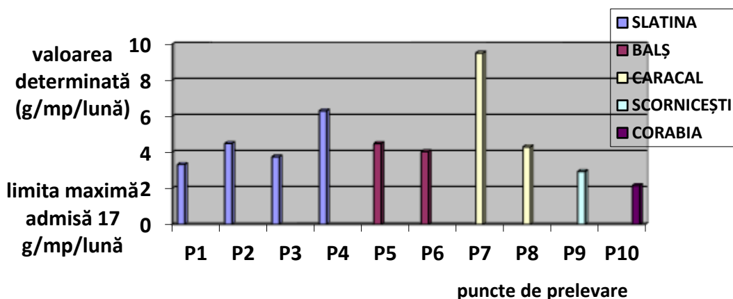
Fig. 1.9. Valori determinate pulberi sedimentabile
