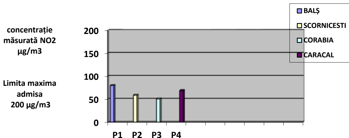
Fig. 1.8. Valori concentrației măsurate NO 2
