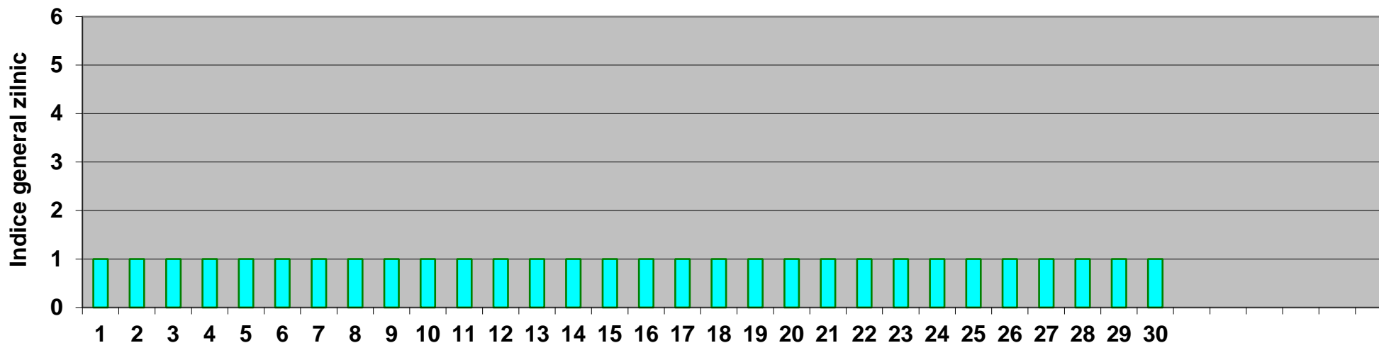
Fig.1.2. Evoluția indicelui general de calitate a aerului în luna NOIEMBRIE 2023 la stația OT-1 (Slatina, Aleea Grădiște F.N.)
