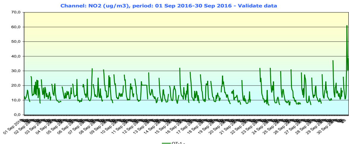
Fig. 1.4 Evoluție valori medii orare \text{NO}_2 la stația automată din județul Olt – luna septembrie 2016
