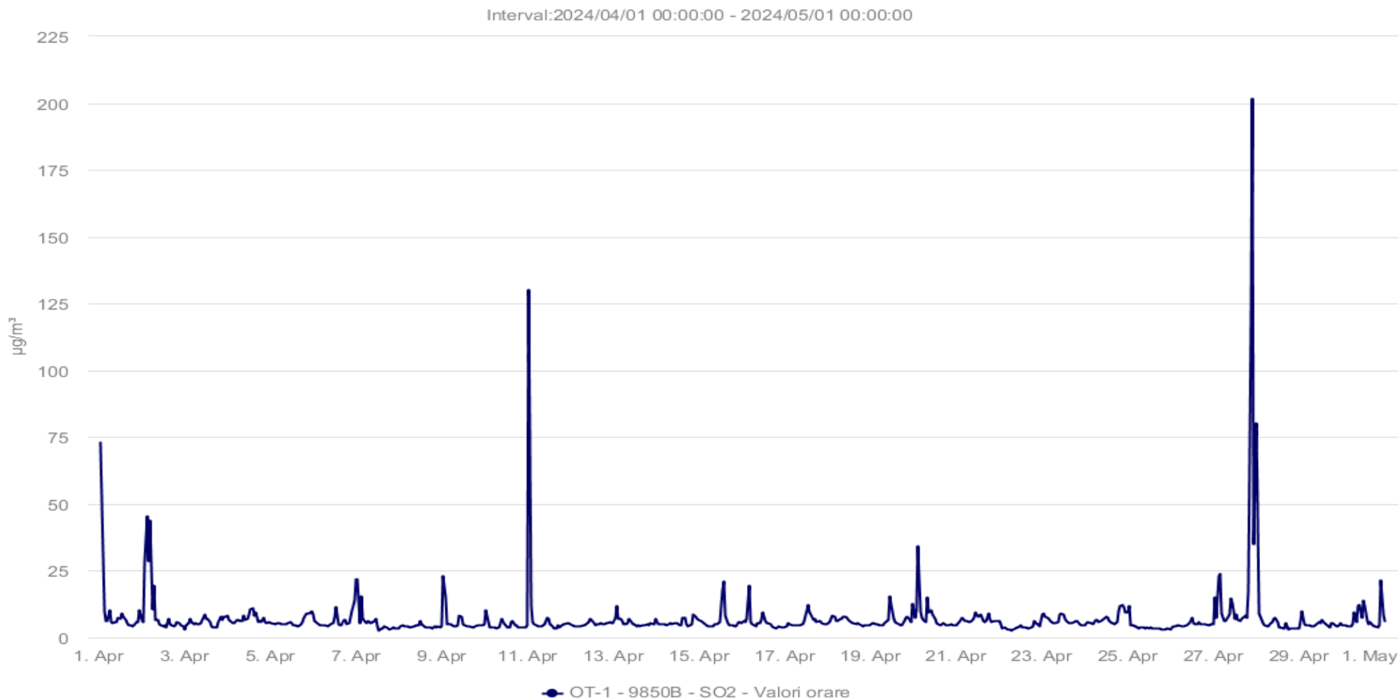
Fig. 1.5. Evoluție valori medii orare \text{SO}_2 la stația automata OT1 din județul Olt - luna APRILIE 2024.
