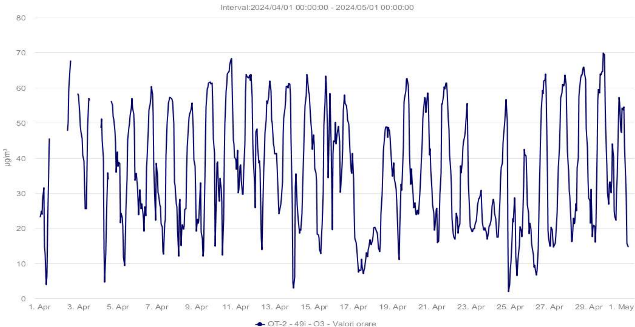
Fig. 1.7. Evoluție valori medii orare pentru O 3 - luna APRILIE 2024
