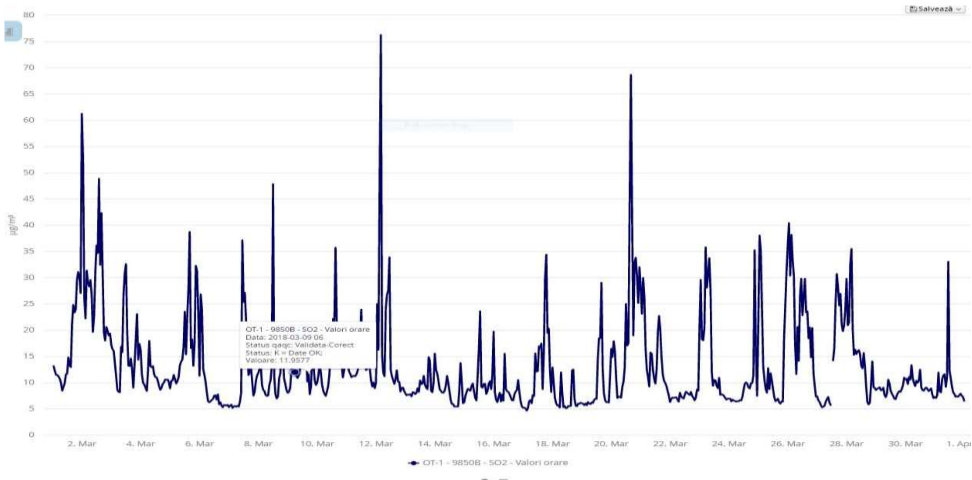
Fig. 1.2 Evoluție valori medii orare SO 2 la stația automata din județul Olt – luna martie 2018.
