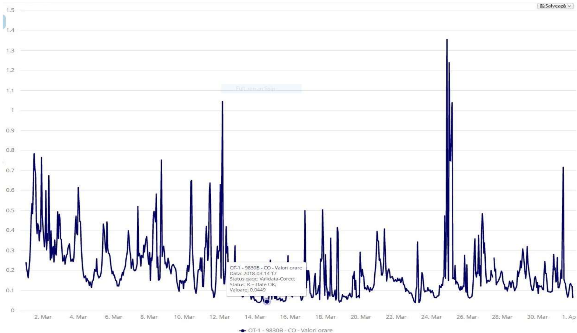
Fig. 1.4 Evoluție valori medii orare pentru CO - luna martie 2018
