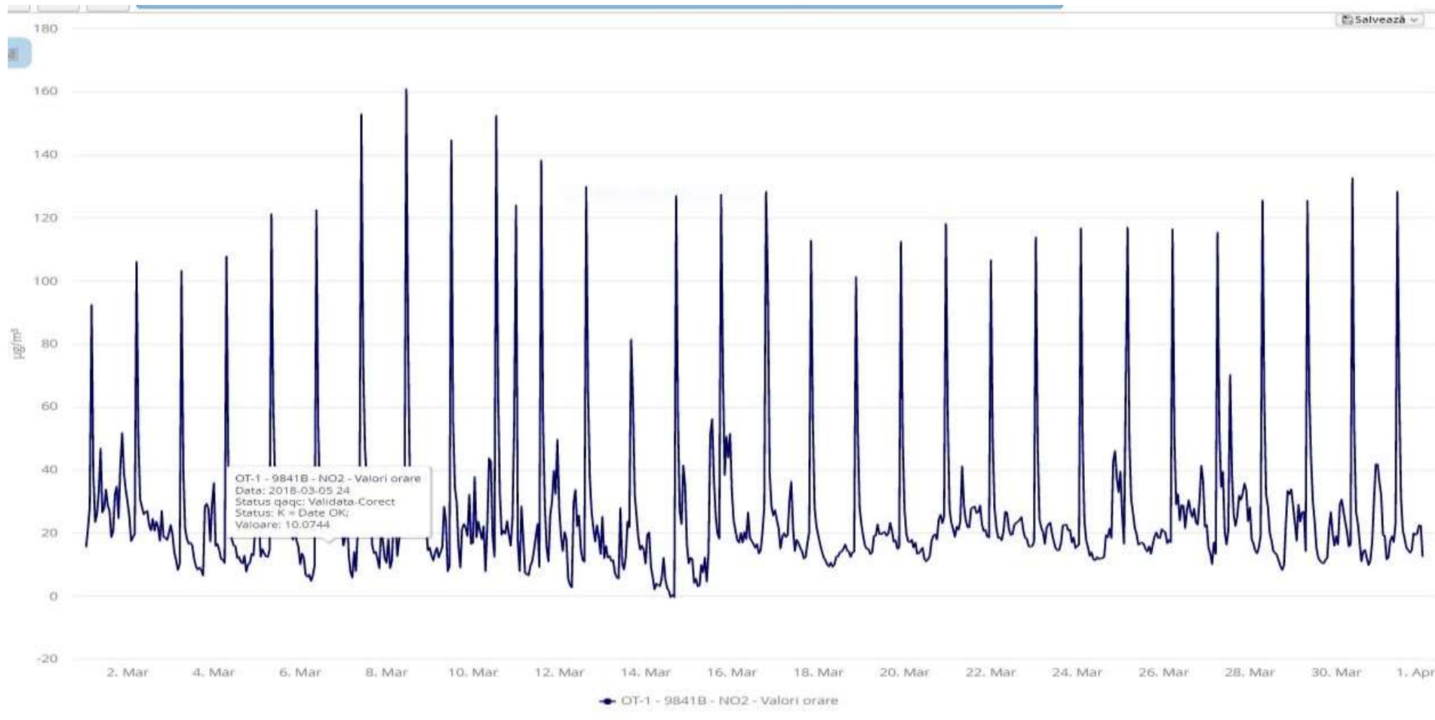
Fig. 1.3 Evoluție valori medii orare NO 2 la stația automată din județul Olt – luna martie 2018
