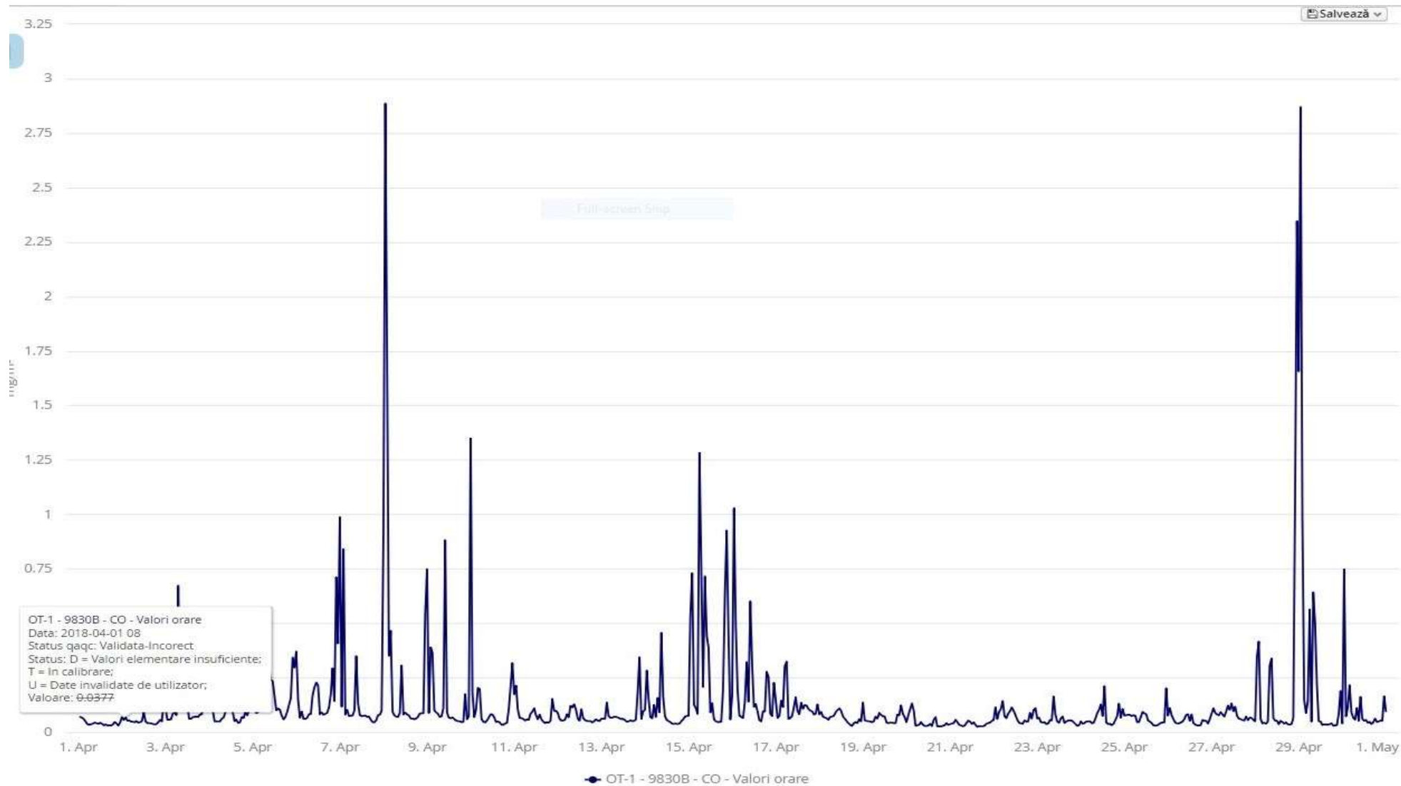
Fig. 1.4 Evoluție valori medii orare pentru CO - luna aprilie 2018
