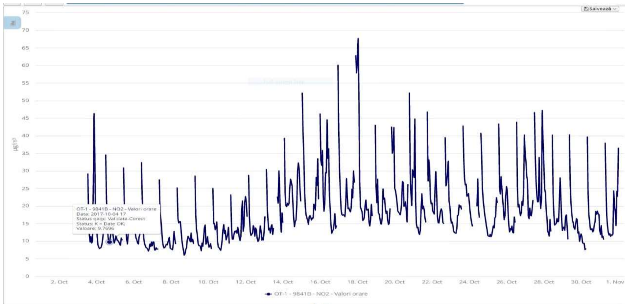
Fig. 1.3 Evoluție valori medii orare NO 2 la stația automată din județul Olt – luna octombrie 2017
