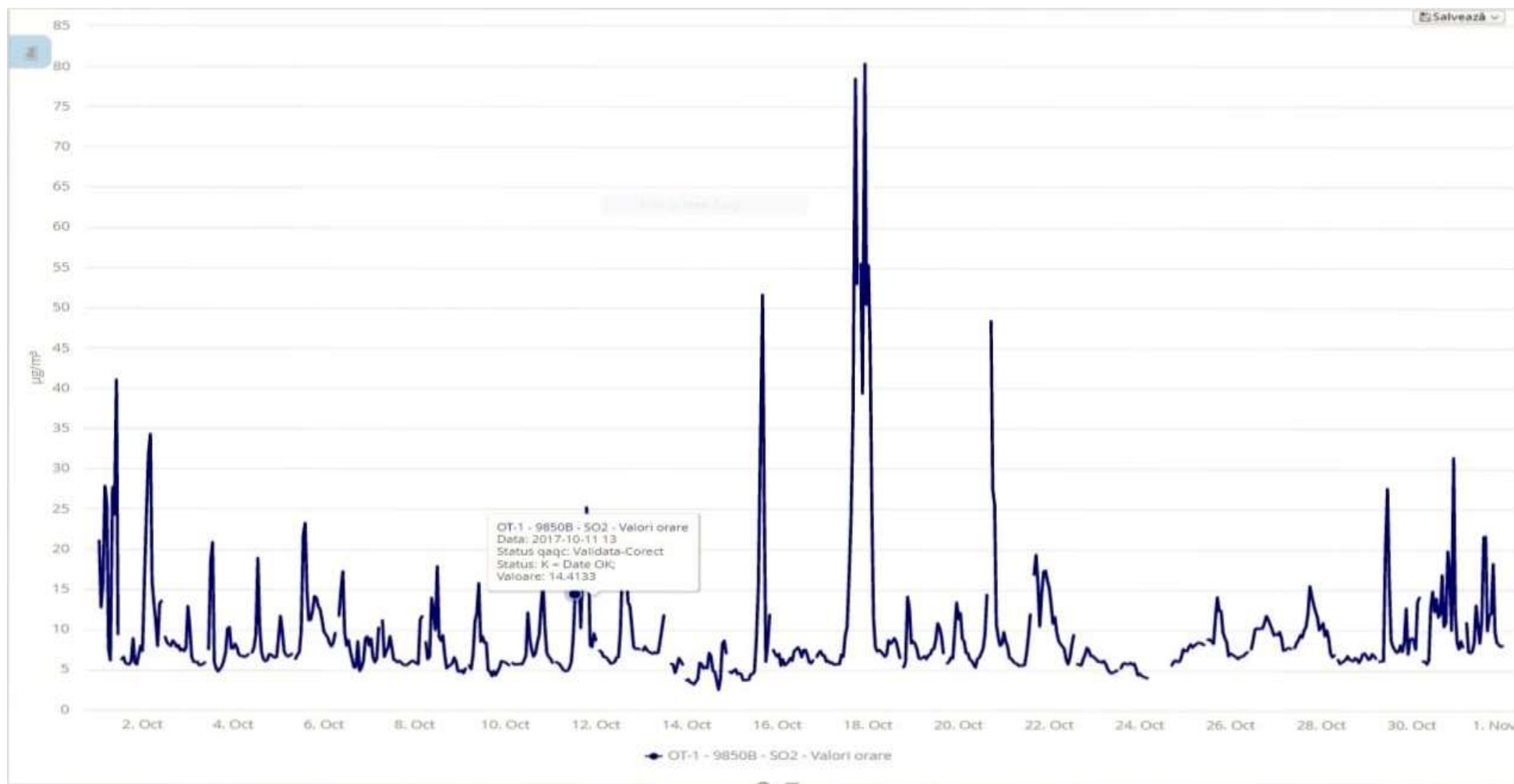
Fig. 1.2 Evoluție valori medii orare SO 2 la stația automata din județul Olt – luna octombrie 2017
