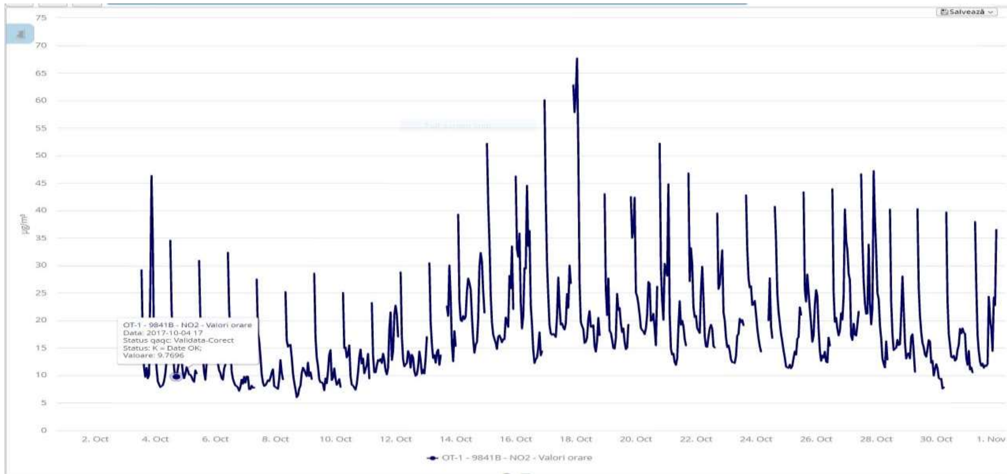
Fig. 1.3 Evoluție valori medii orare \text{NO}_2 la stația automată din județul Olt – luna octombrie 2017
