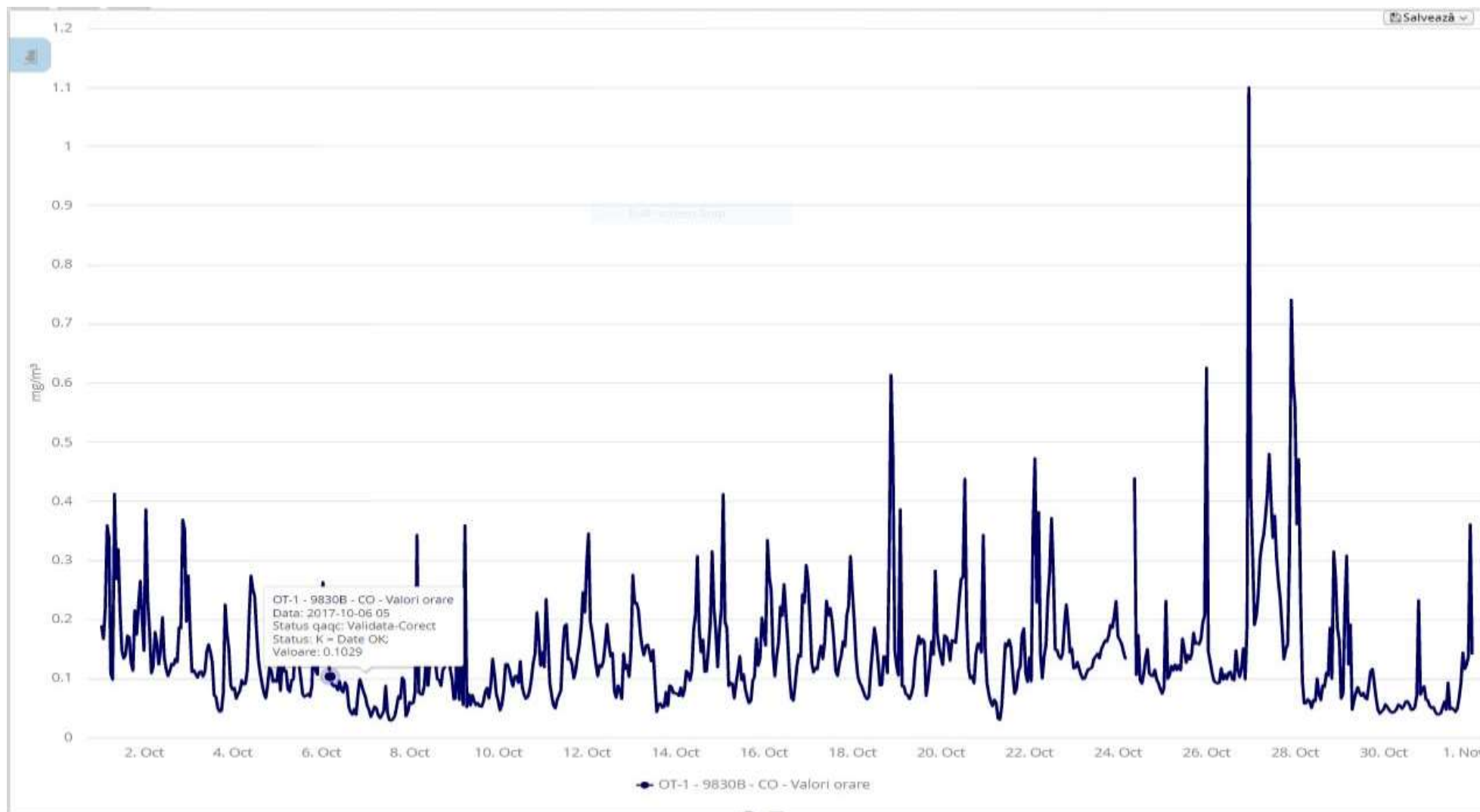
Fig. 1.4 Evoluție valori medii orare pentru CO - luna octombrie 2017
