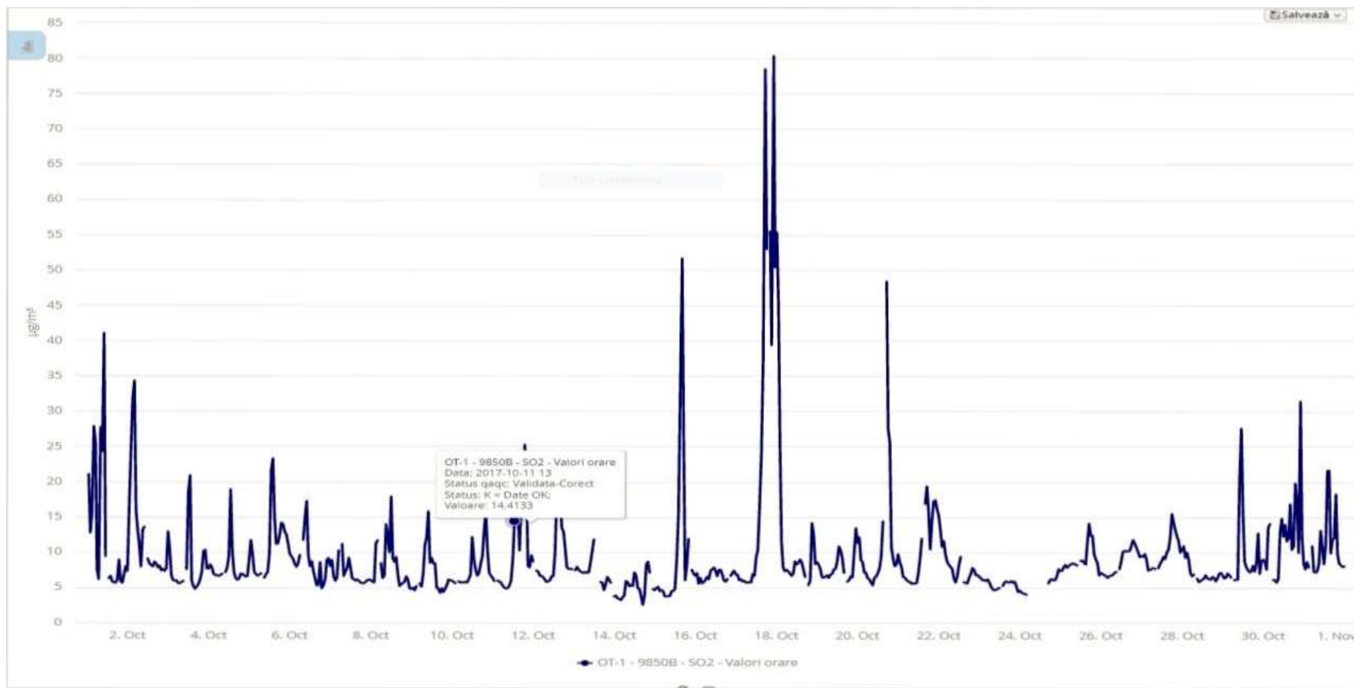
Fig. 1.2 Evoluție valori medii orare SO 2 la stația automata din județul Olt – luna octombrie 2017
